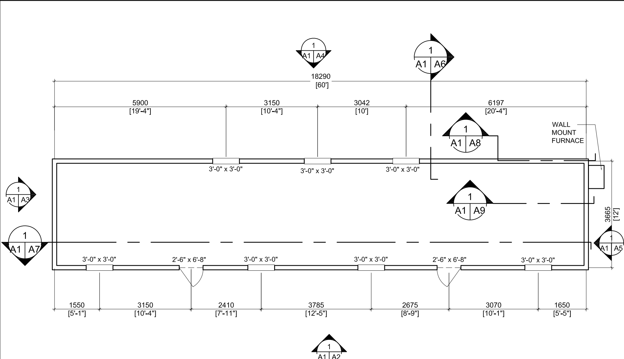
1 FLOOR PLAN A1 | A1 1:80 M
