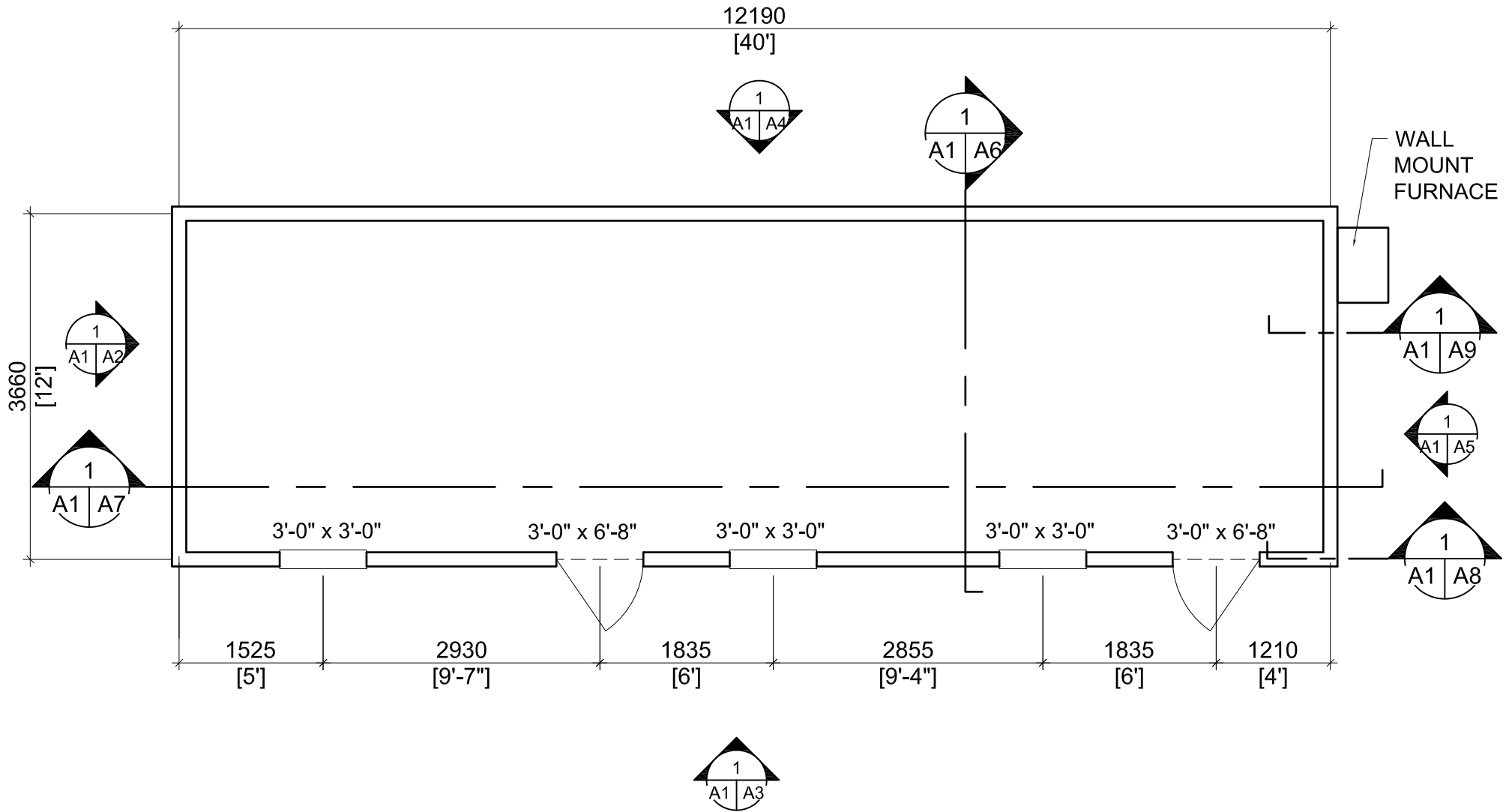
1 FLOOR PLAN A1 | A1 1:60 M
